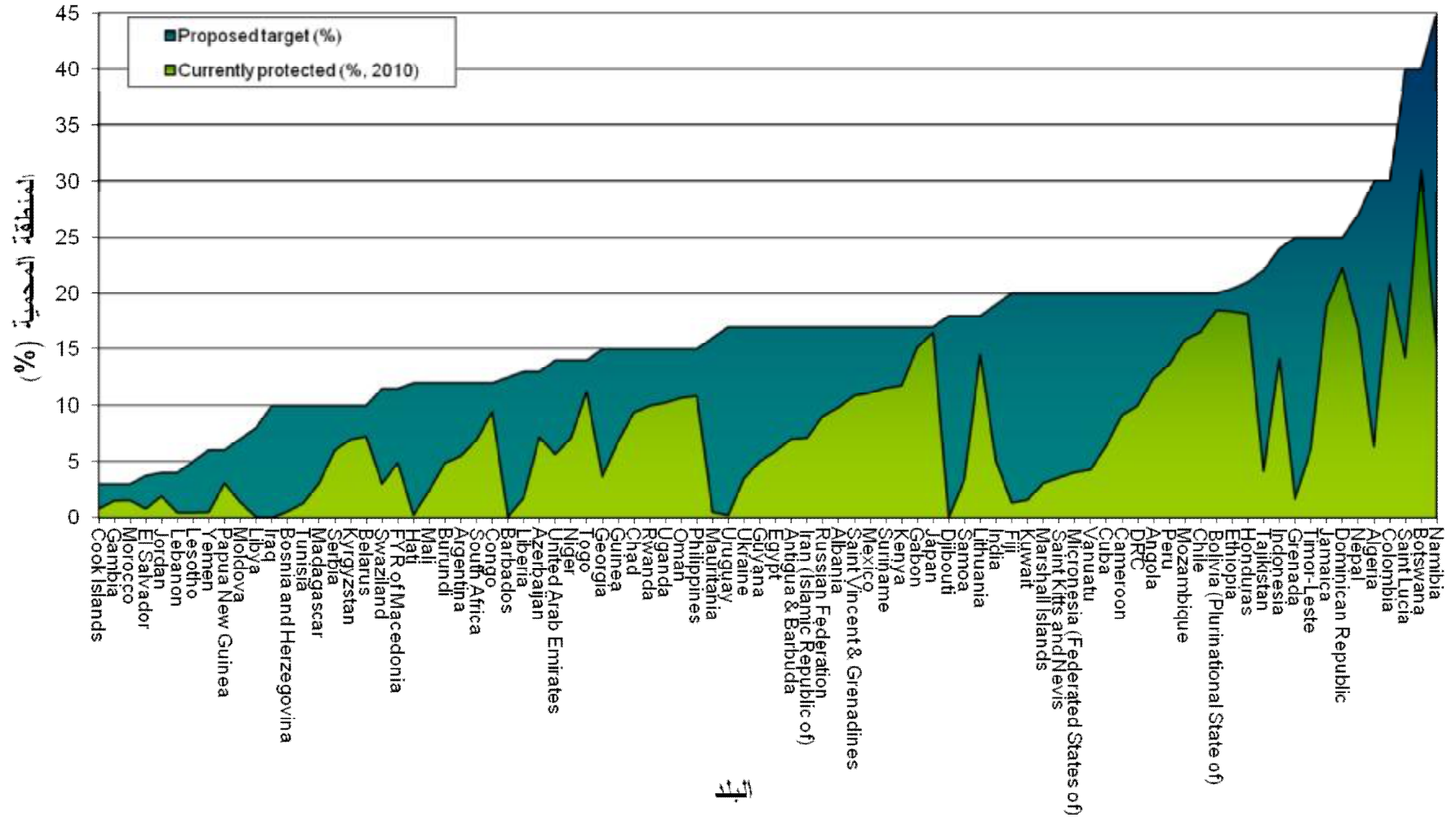
الشكل 2 - النسبة المئوية الحالية والمستهدفة للمناطق الأرضية الخاضعة للحماية بالنسبة لـ 86 بلدا (المصدر: حلقات عمل بناء القدرات في اتفاقية التنوع البيولوجي وقاعدة البيانات العالمية للمناطق المحيية لعام 2011)
