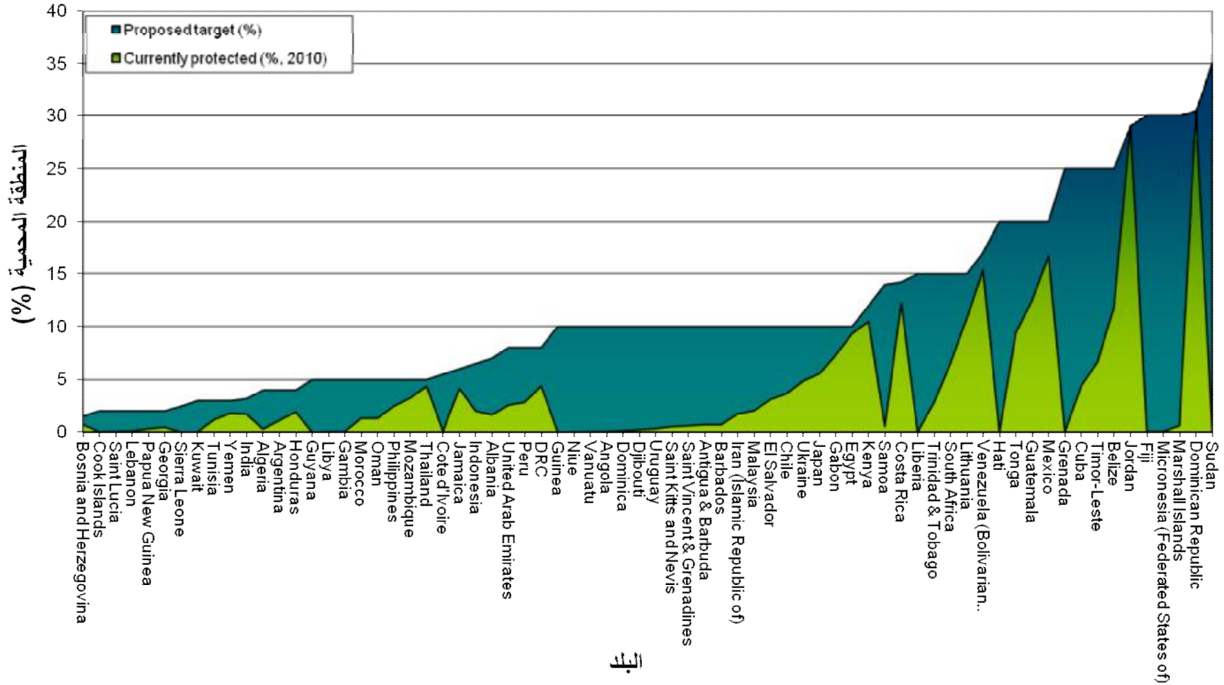
الشكل 3 - النسبة المئوية الحالية والمستهدفة للمياه الإقليمية الخاضعة للحماية بالنسبة لـ 70 بلدا (المصدر: حلقات عمل بناء القدرات في اتفاقية التنوع البيولوجي للسنتين 2011-2012 وقاعدة البيانات العالمية للمناطق المحمية لعام 2011)
